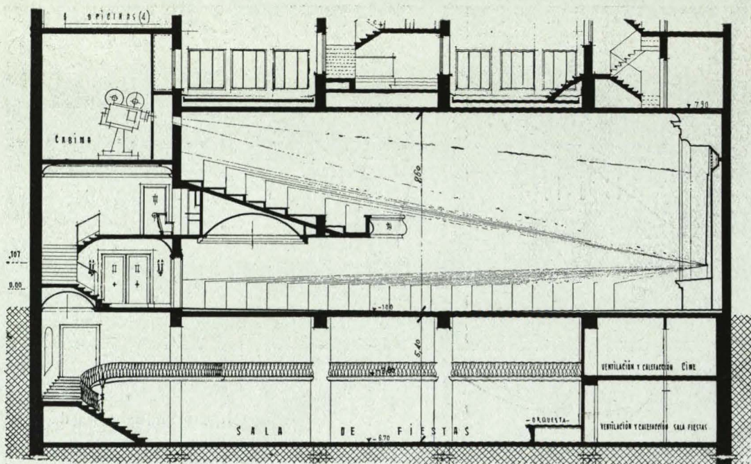
Sección longitudinal.
